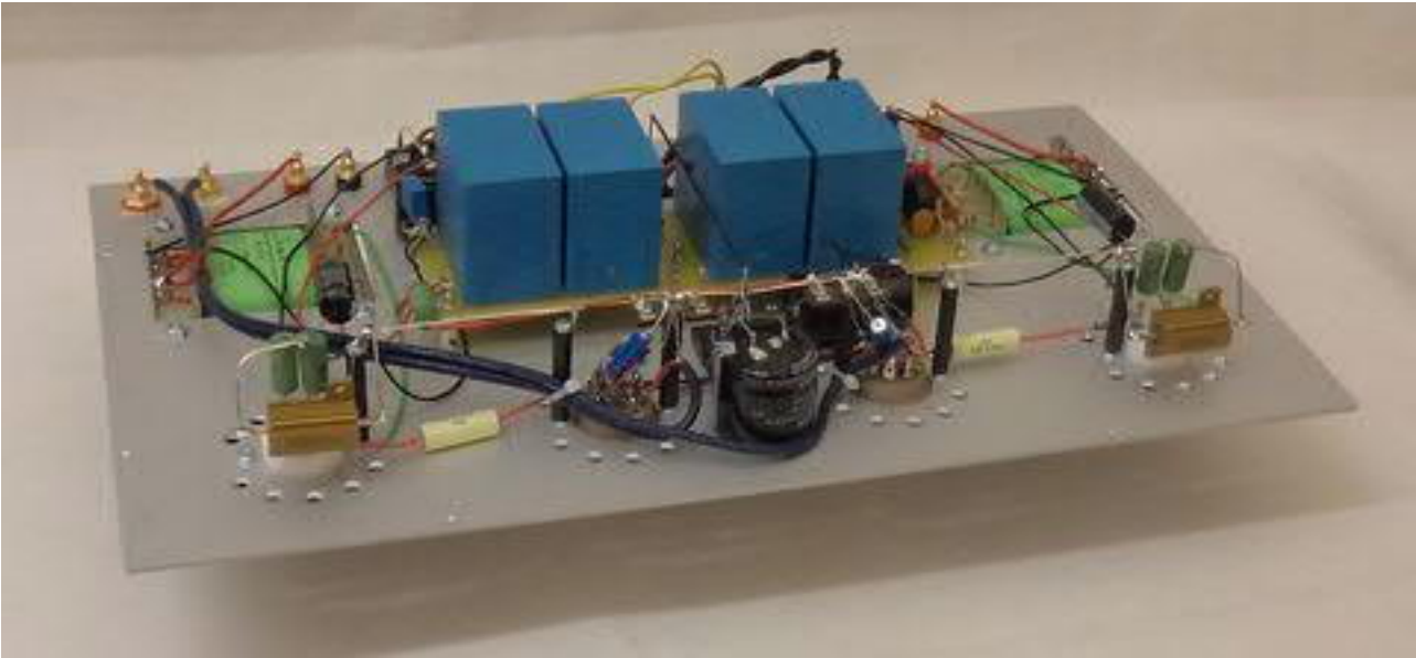
Das nächste Bild zeigt die klassische Handverdrahtung der Endstufe
